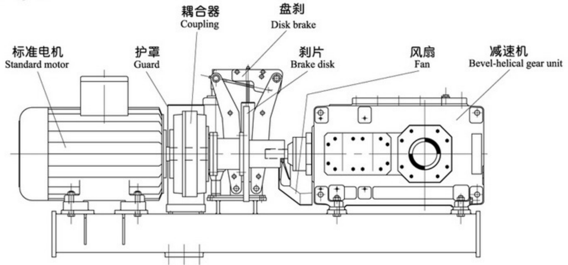
带齿轮箱摆动底座 Gear unit swing-bases
